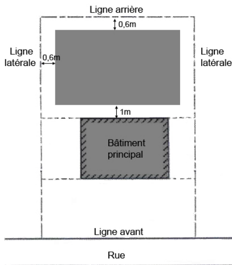
Croquis 9: Antenne numérique / parabolique
