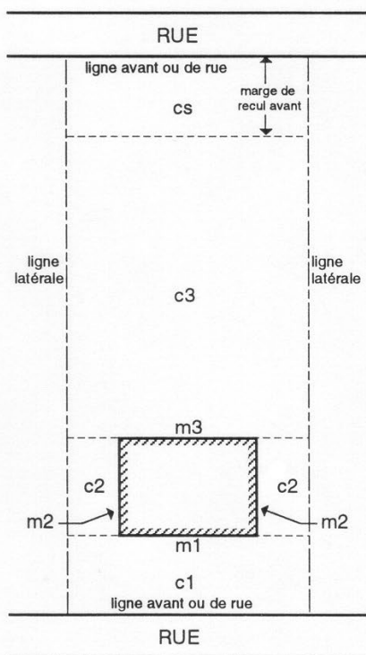
e) Terrain intérieur transversal
