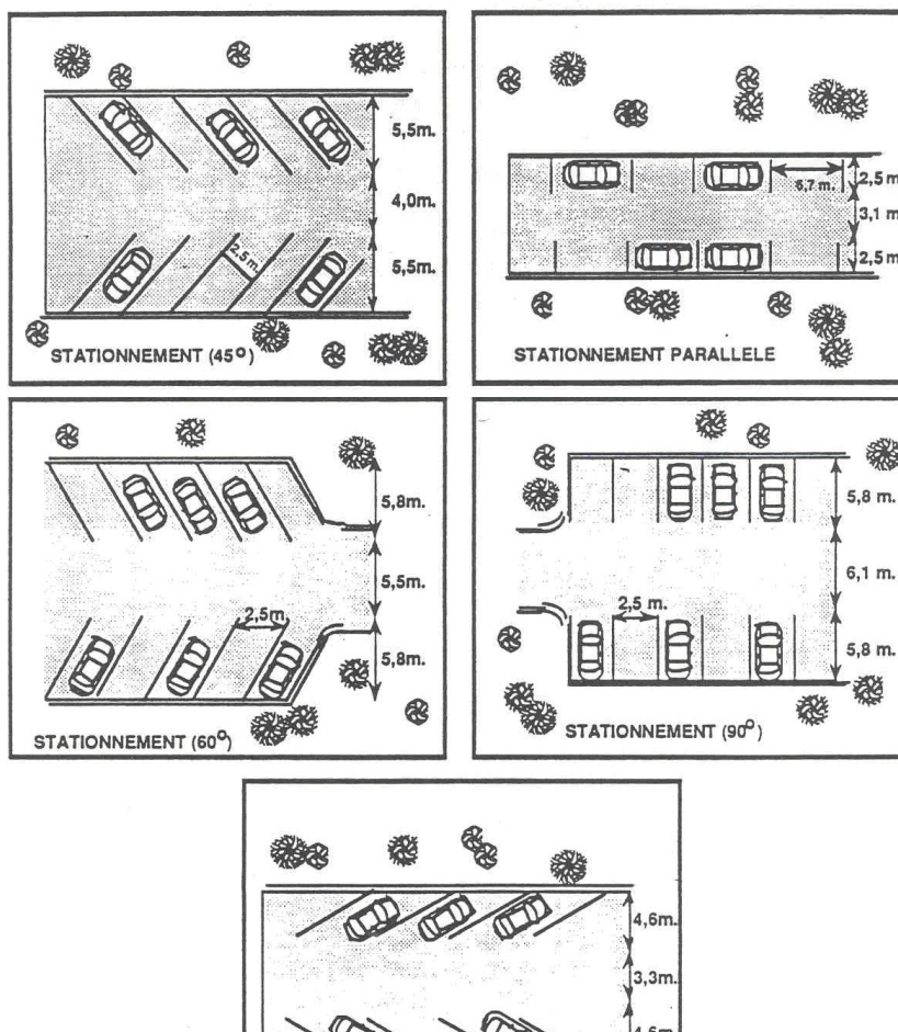
Croquis 66 : Dimension d'une case de stationnement
